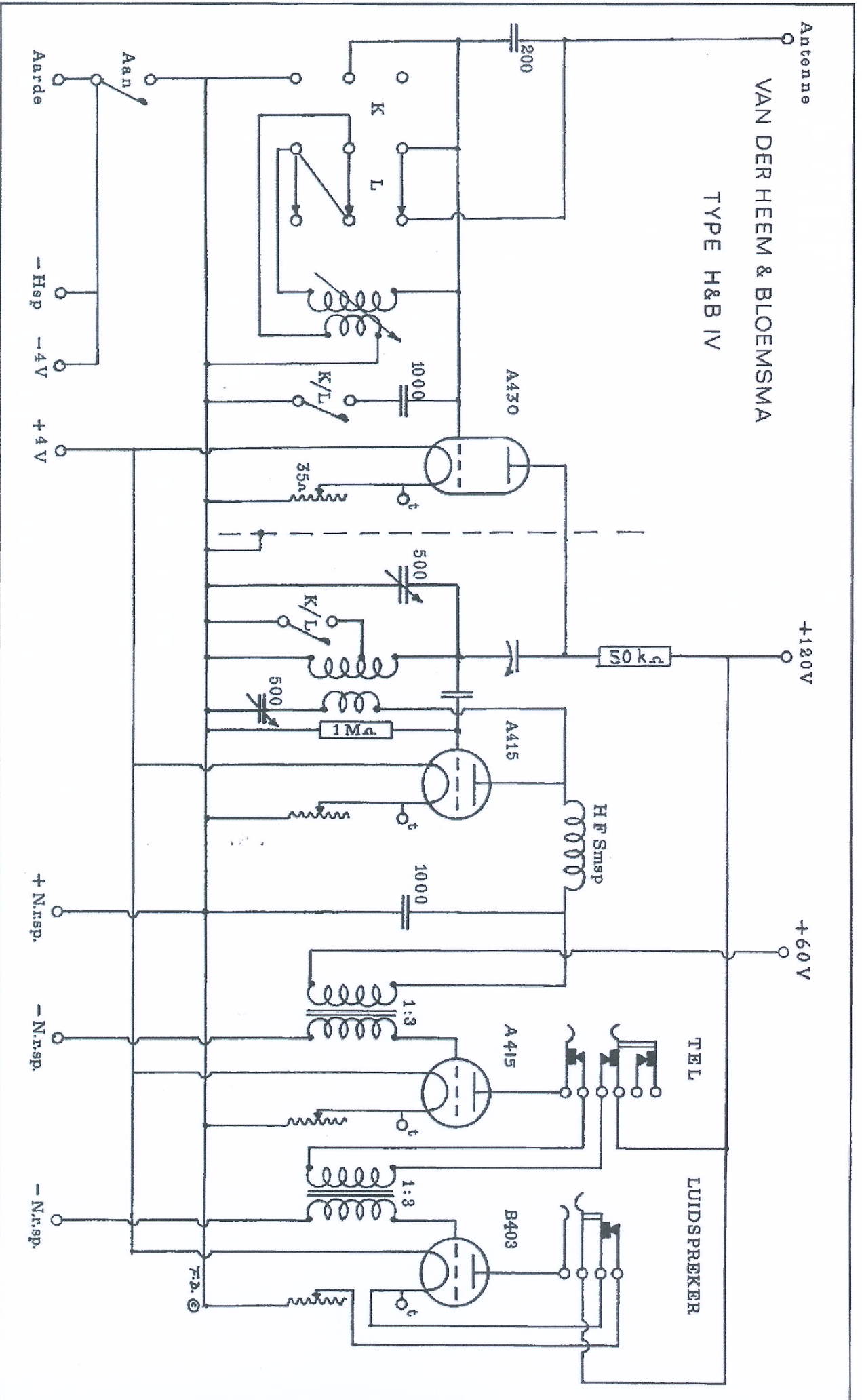
Schema H&B IV 2e uitvoering, februari 1927
